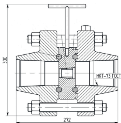
Рис. 2. Схема фланцевого крепления штуцеров
