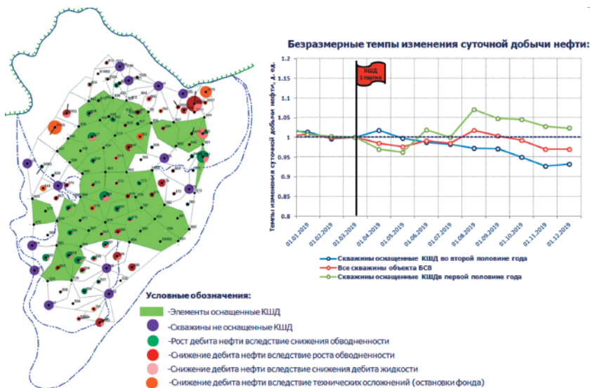
Рис. 6. Эффективность внедрения оборудования КШД
